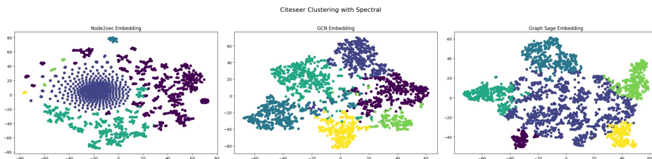
Σχήμα 9: Αποτελέσματα Clustering Spectral για το Citeseer
