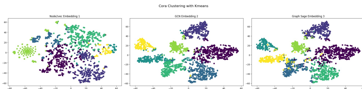
Σχήμα 5: Αποτελέσματα Clustering kmeans για το Cora
