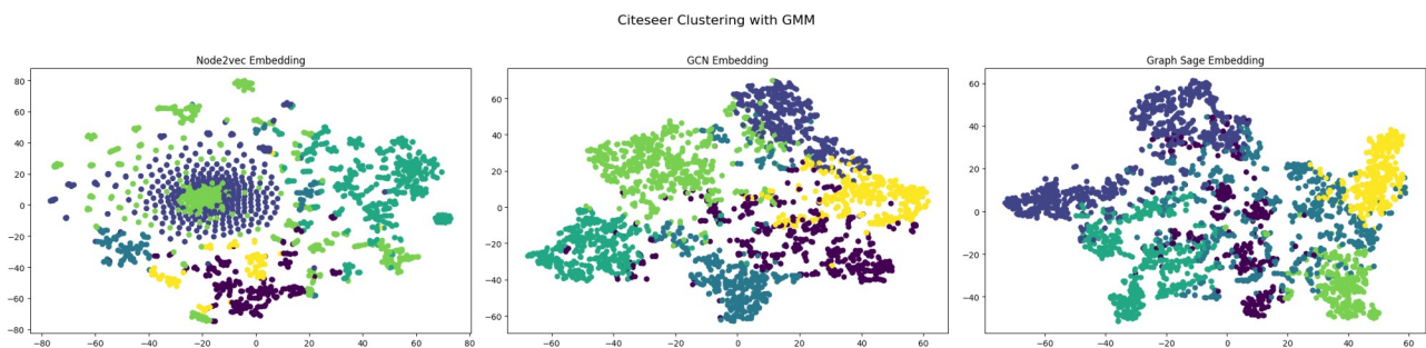
Σχήμα 12: Αποτελέσματα Clustering GMM για το Citeseer
