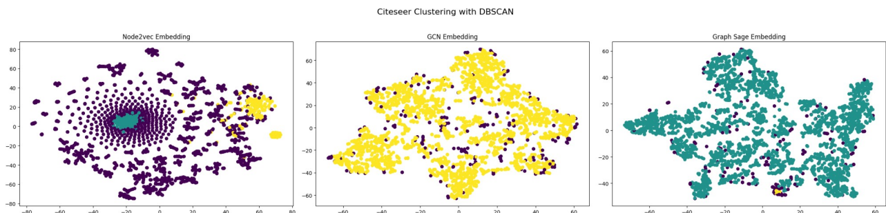
Σχήμα 8: Αποτελέσματα Clustering DBSCAN για το Citeseer
