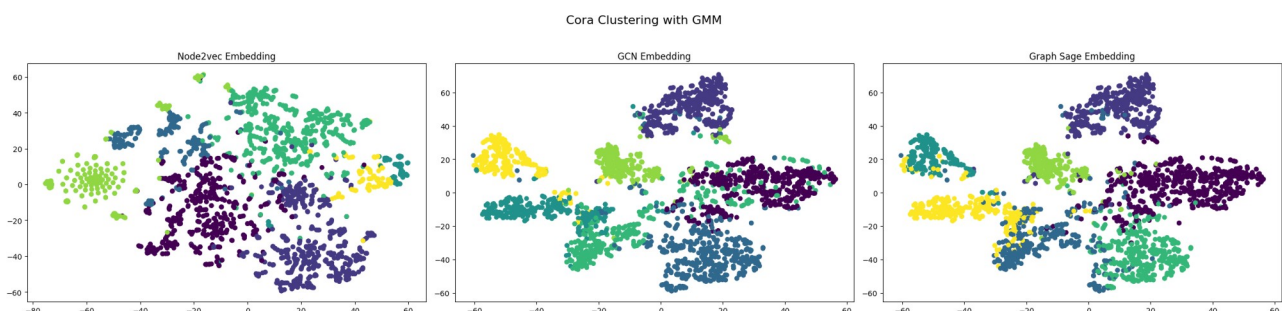
Σχήμα 11: Αποτελέσματα Clustering GMM για το Cora
